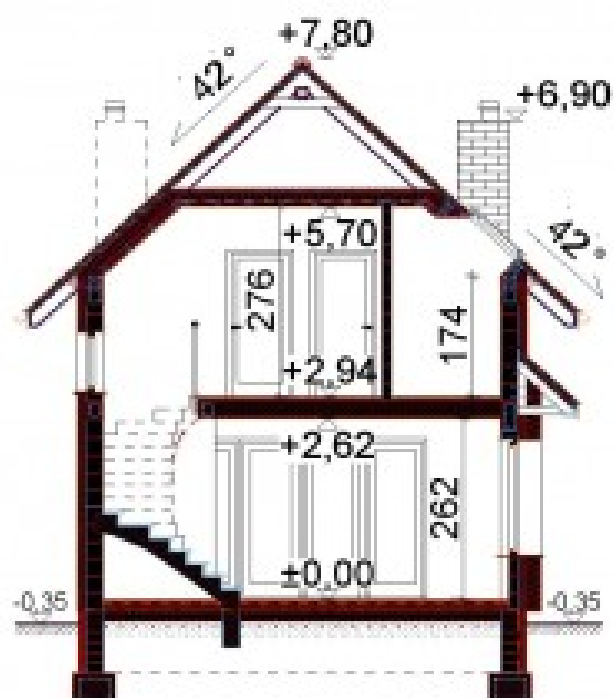
PRZEKRÓJ A-A
